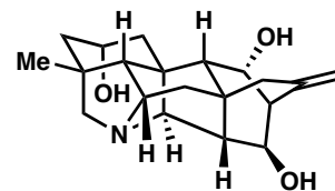
Hetisine
